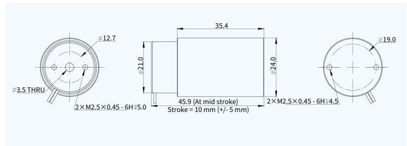
■ 尺寸图
