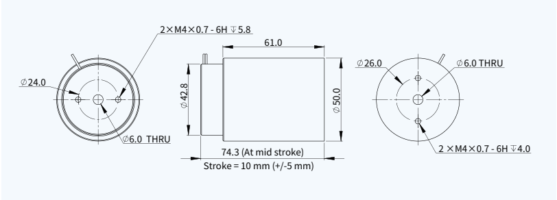
尺寸图
