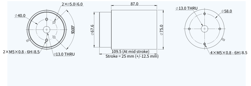
■ 尺寸图
